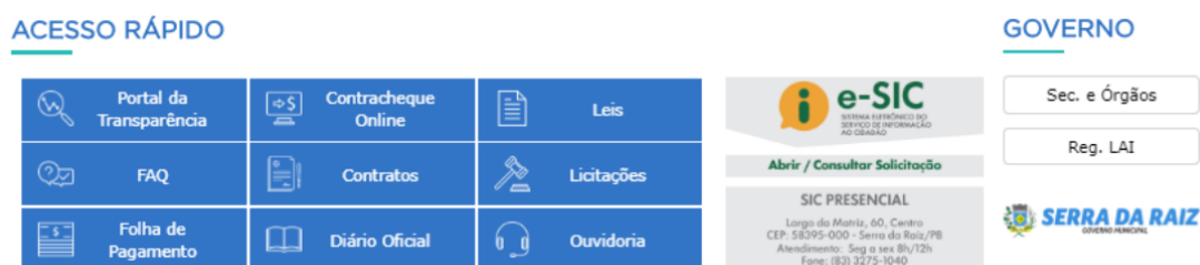
Figura 6 - Acesso rápido
