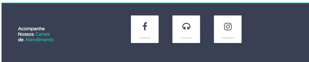
Figura 7 - Redes sociais
